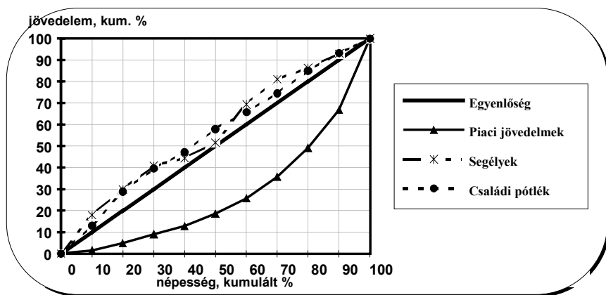
6.c ábra A piaci jövedelmek és a szociális támogatások elosztási mintái: Lorenz-görbék 1995/96-ra
